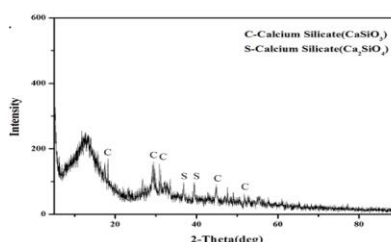
高壓蒸煮後試體XRD分析
